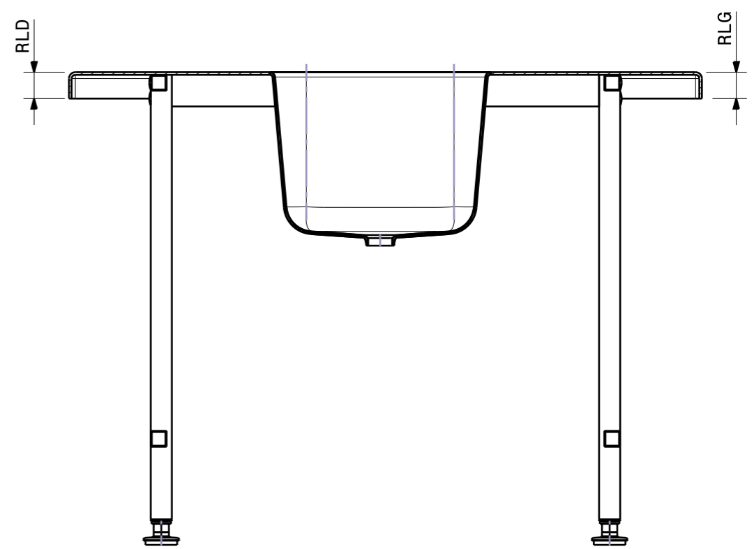
Coupe B-B Echelle : 1:10
